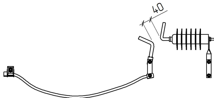
Комплект захисту ПЛЗ від атмосферних перенапруг ASIC 300u поз. 11
